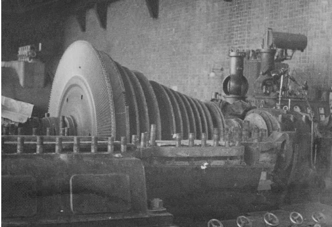
Turbine 1 im Peenemünder Kraftwerk nach einem Schaden am Läufer der 12. Stufe im Jahre 1966 Foto: HTM Peenemünde, Archiv
